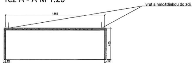
řez A - A' M 1:20
