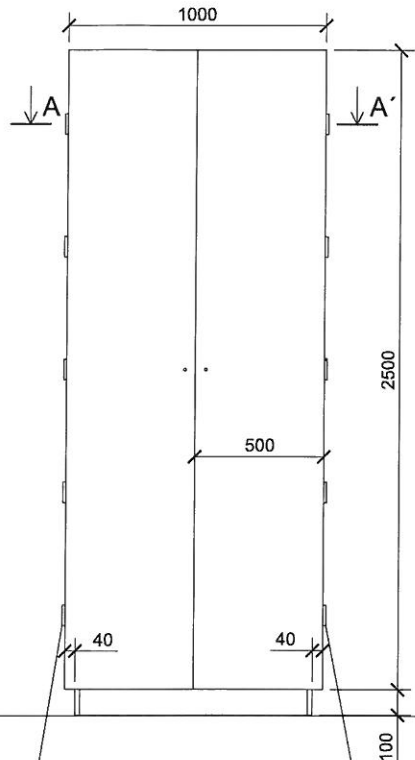
nárys M 1:20
