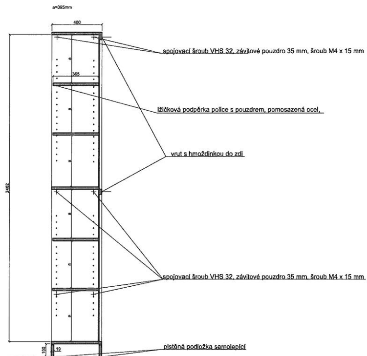
řez B-B' M 1:20
