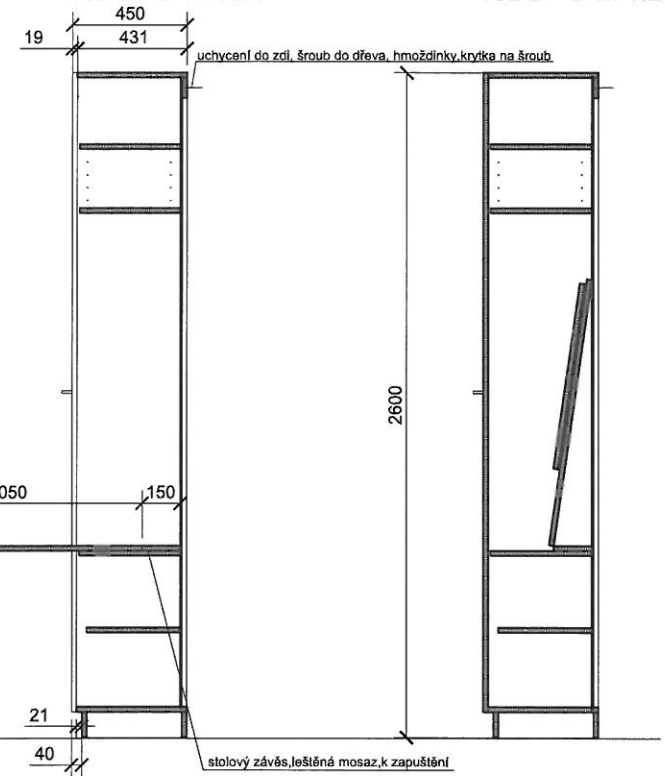
řez B - B' M 1:20
