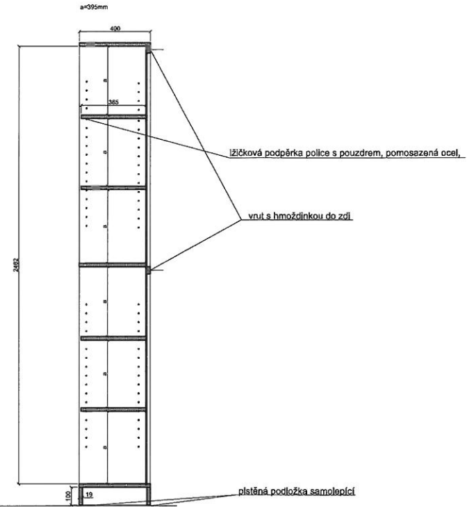
řez B-B' M 1:20
