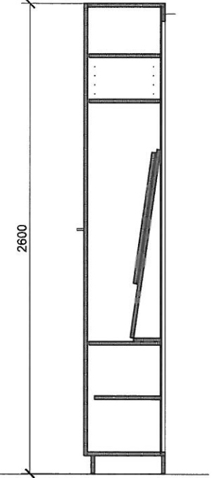
řez B - B' M 1:20
