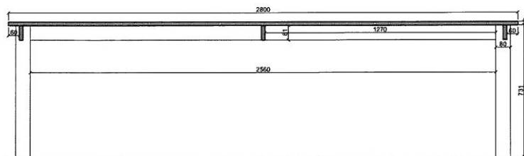
řez C - C' M 1:20
