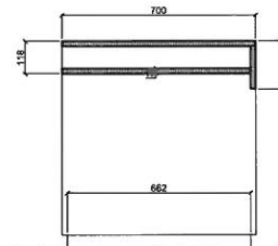
řez C - C'M 1:20
