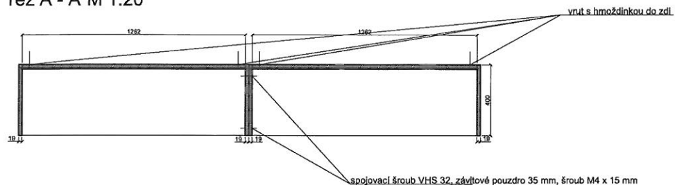
řez A - A' M 1:20
