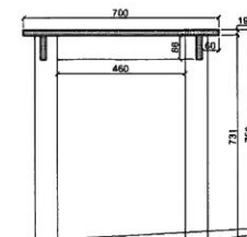
řez B-B' M 1:20
