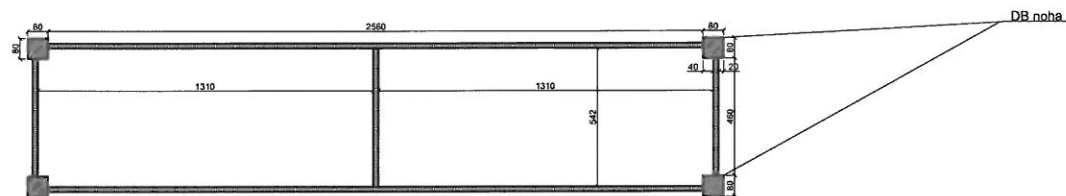
řez C - C' M 1:20
